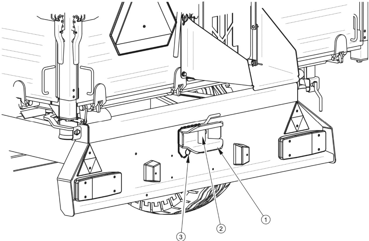
ABBILDUNG 4.2 Hintere Anhängerkupplung
