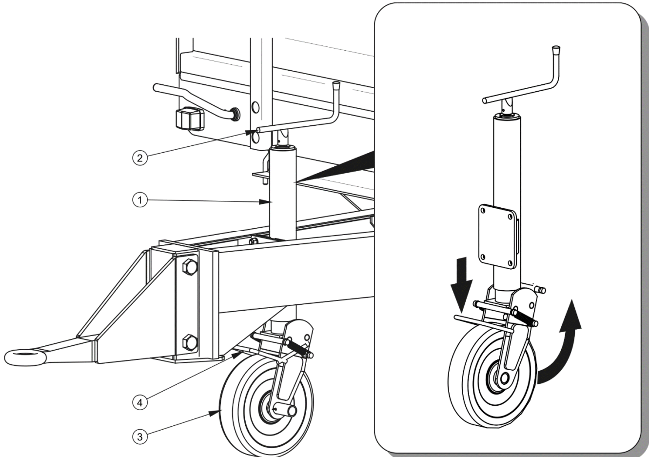
ABBILDUNG 4.1 Anhängerstütze
